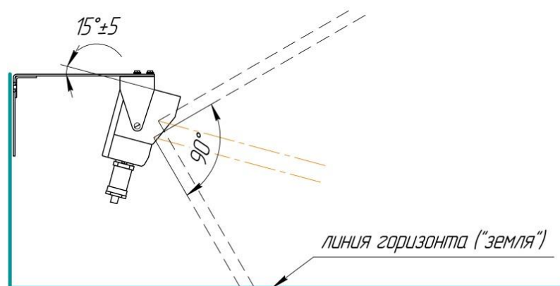
Правильное ориентирование
