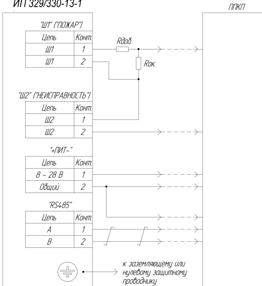
Рисунок А.1 – Схема подключения извещателя по 4- проводному шлейфу
