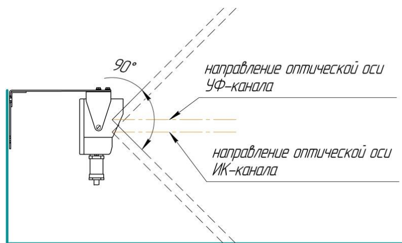
Неправильное ориентирование
