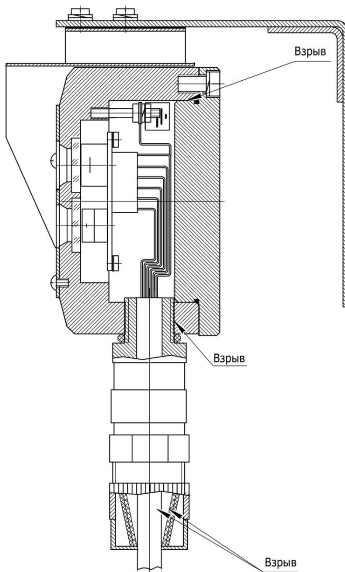
Рисунок 4 – Защита от коррозии
